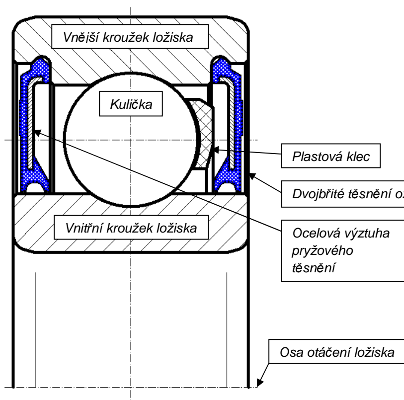
Obrázek polovičního průřezu ložiskem 608-2RZTNH
